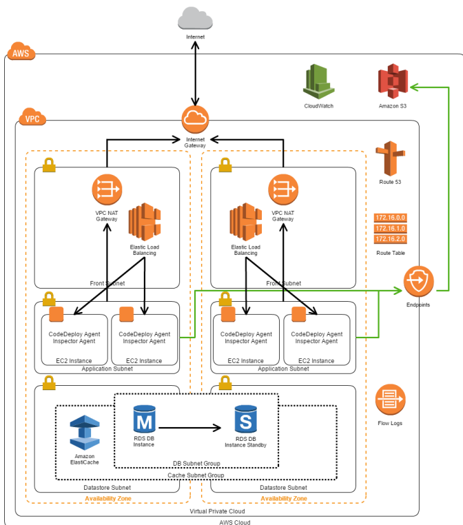
プライベートネットワーク構成
