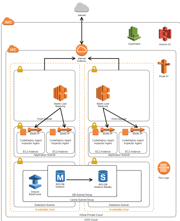
パブリックネットワーク構成
